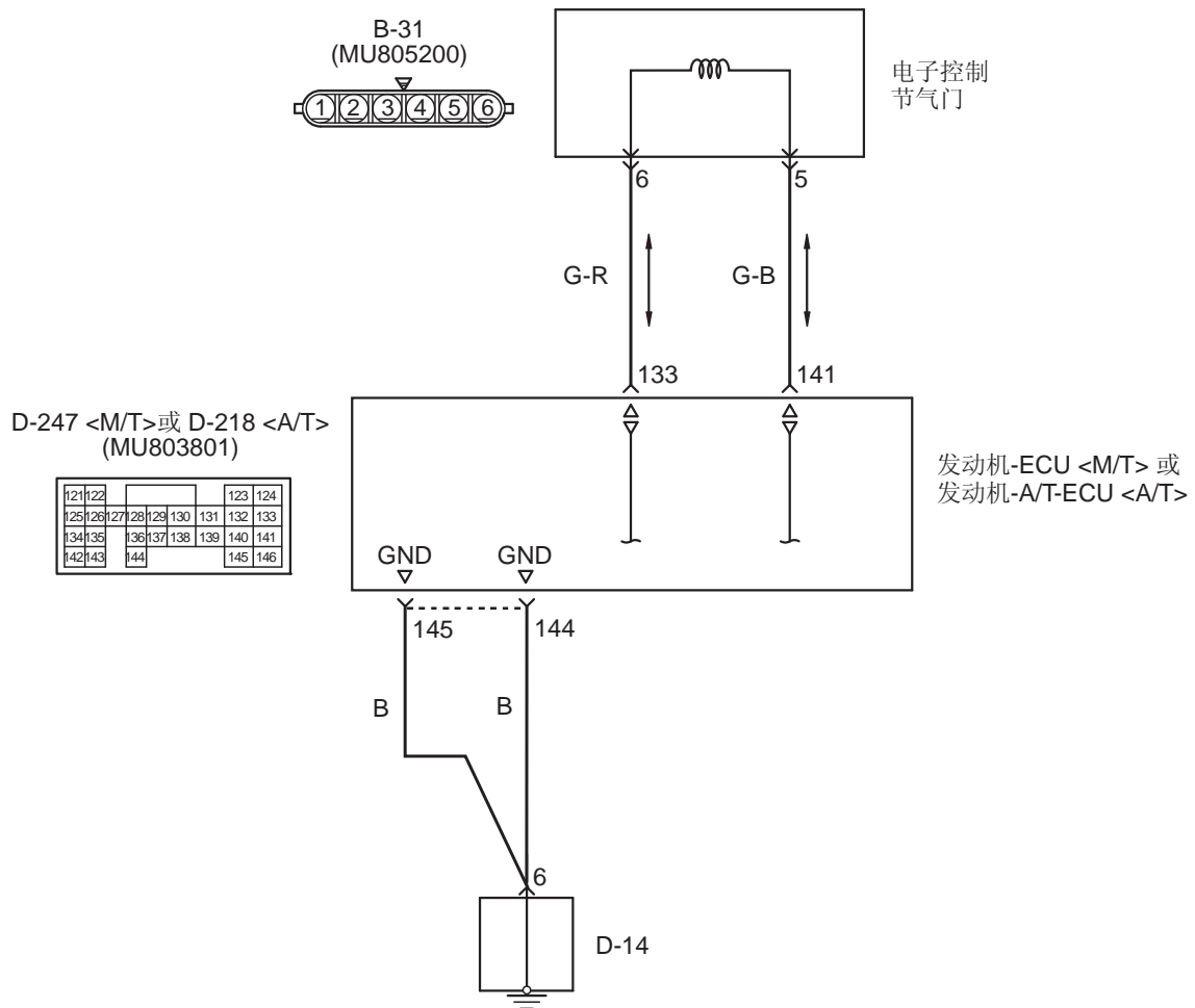
节气门控制伺服电路
